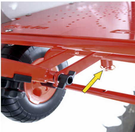
Klappsplint an der Lenkung unten entfernen put off the linch pin of the steering
