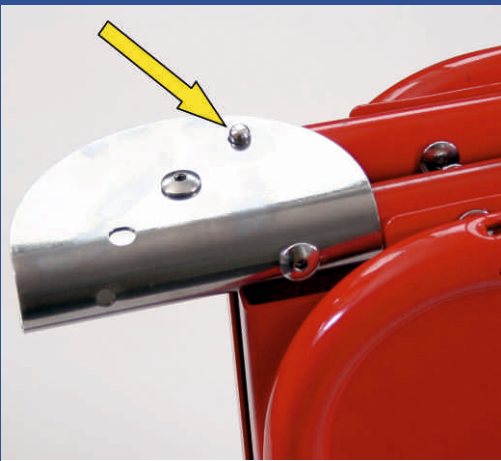
Stellen Sie sicher dass der Rastknopf eingearstet ist. Make sure that the snap button is locked.
